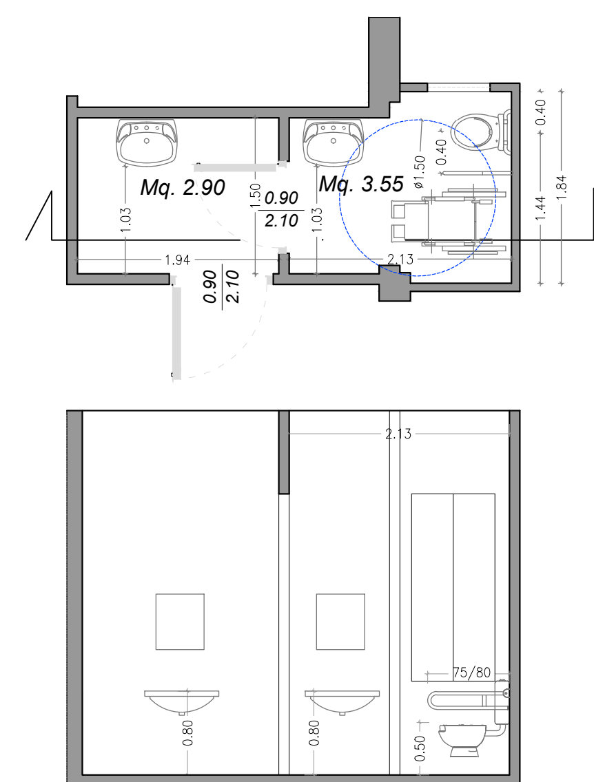
Particolare bagno Sc. 1:50
