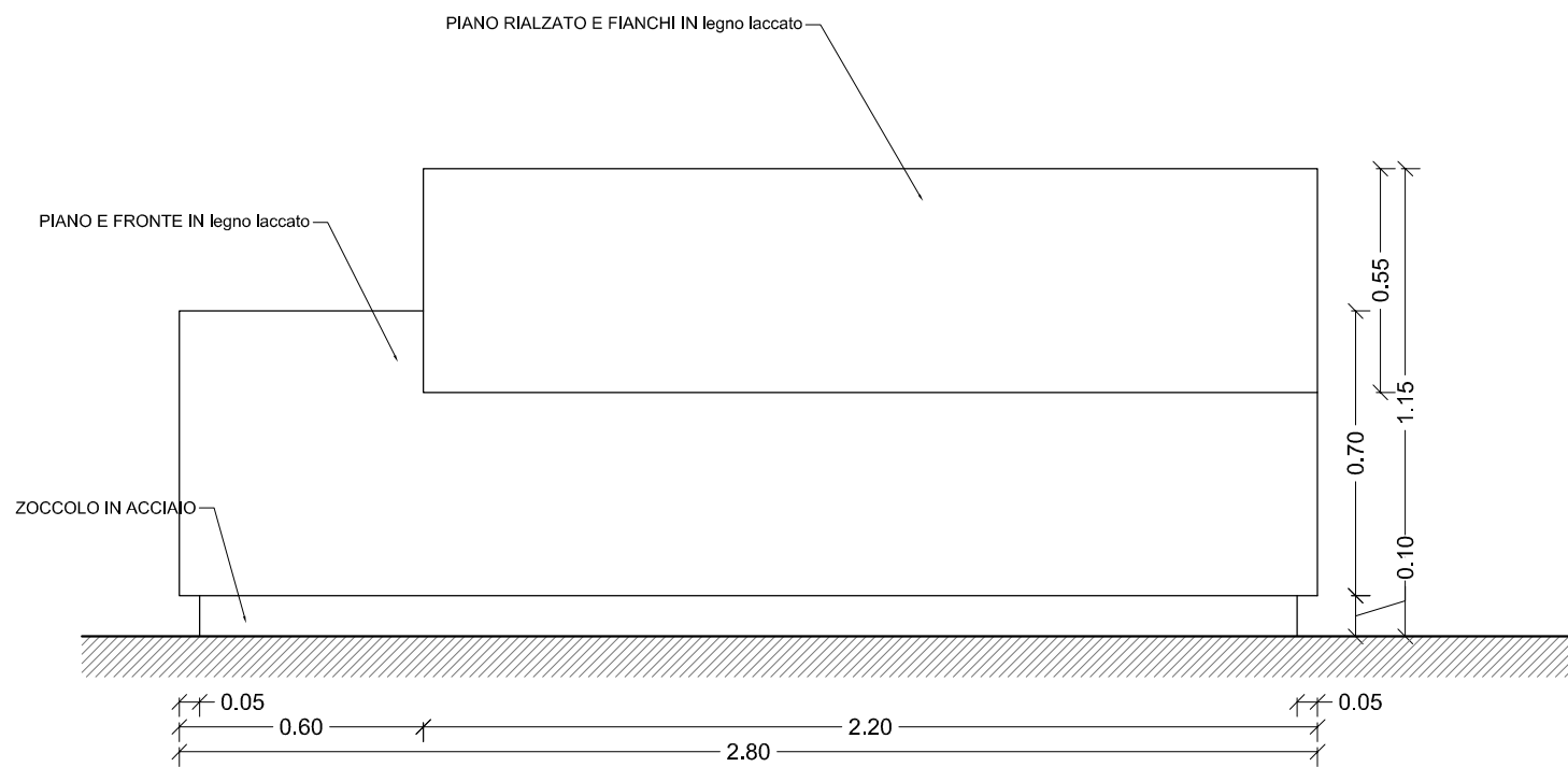
1 | PIANTA 3 | PROSPETTO FRONTALE
